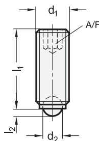
Typ A / AN
